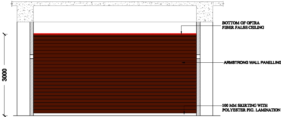
ELEVATION - D
