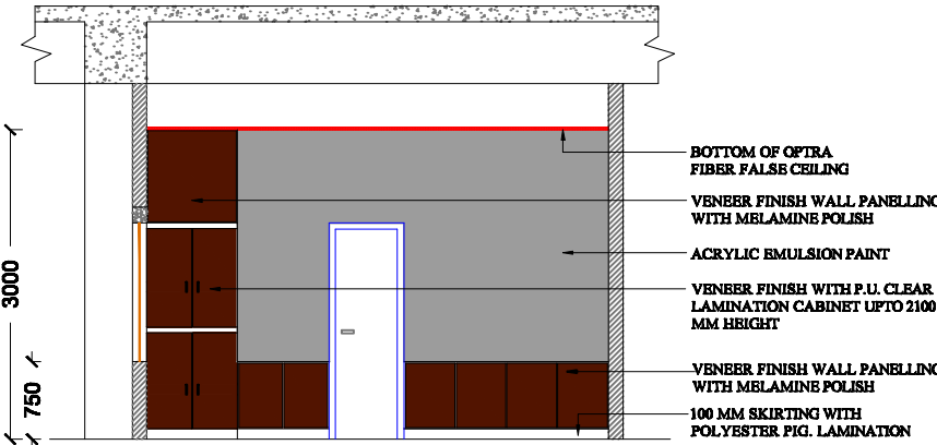
ELEVATION - C
