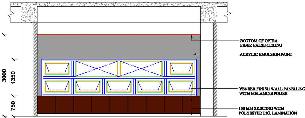
ELEVATION - B
