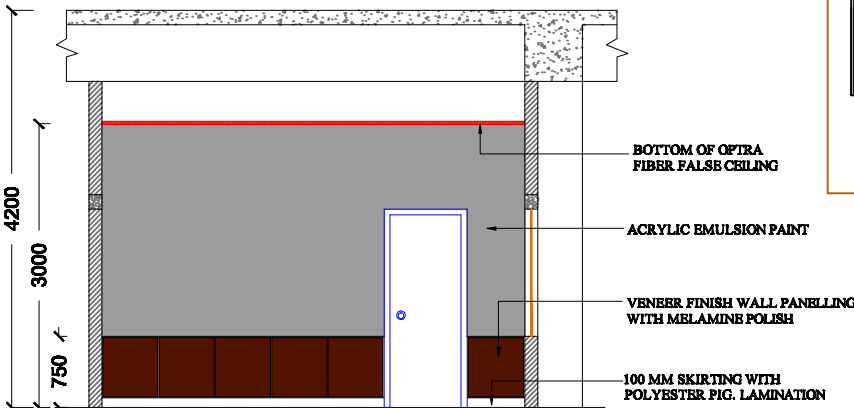
ELEVATION - A
